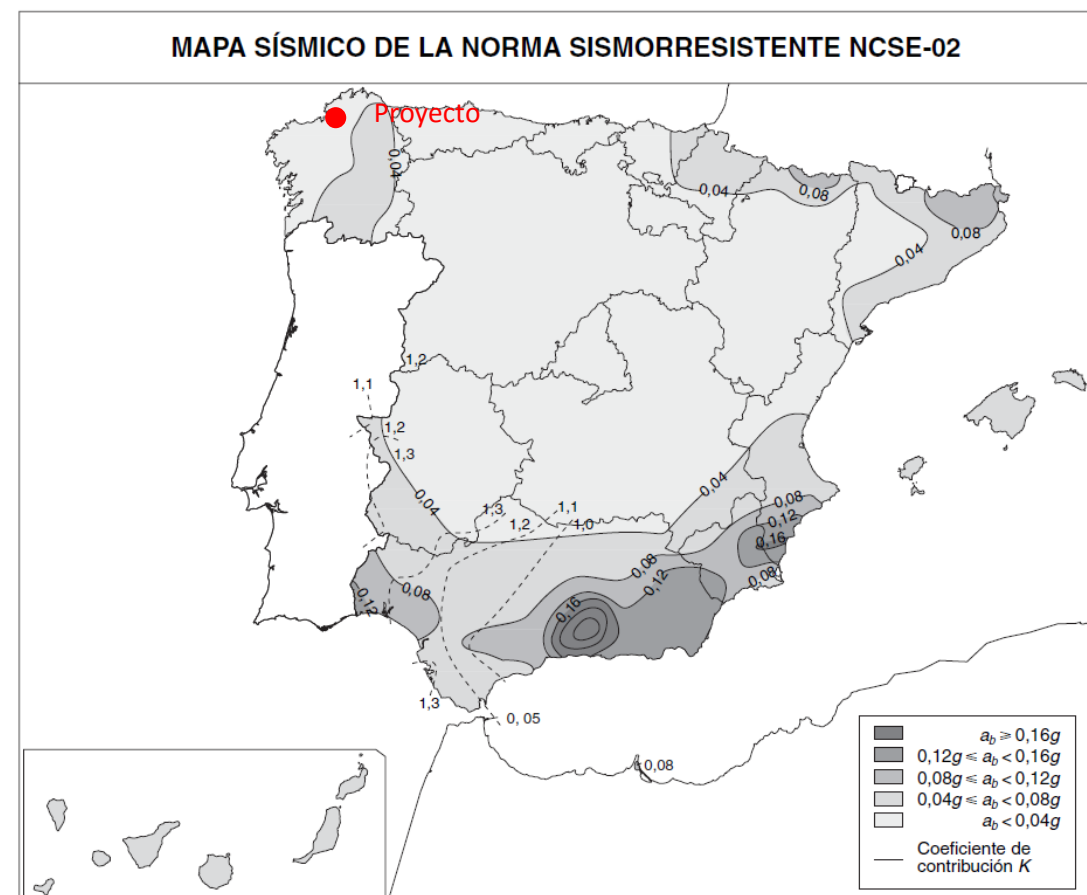
Figura 1. Mapa de peligrosidad sísmica (según NCSE-02 / NCSP-07)
