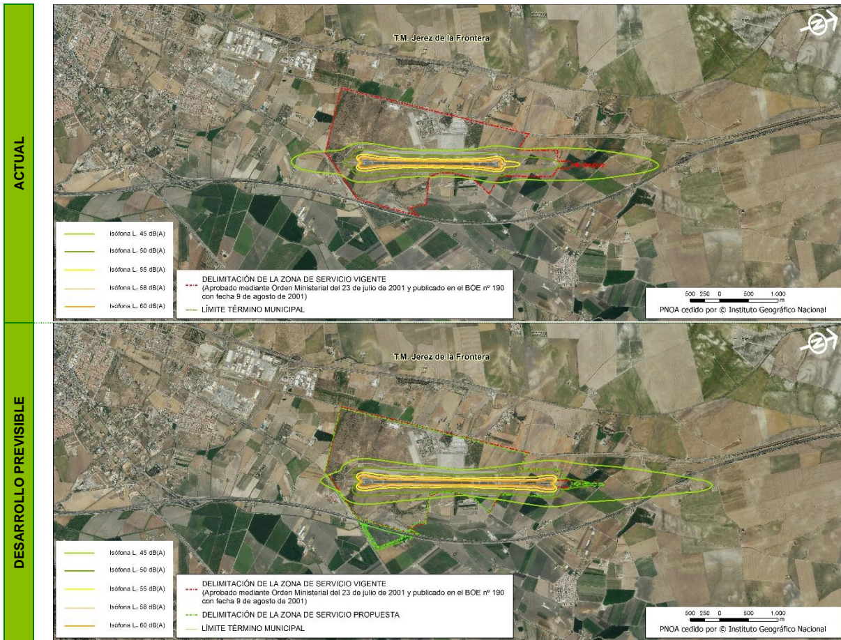
Ilustración III.23.- Huellas acústicas del aeropuerto de Jerez. Periodo noche (23-7h).
