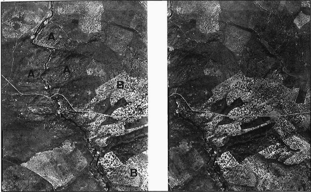
Figura 3.22.- Vista estereoscópica de un berrocal granítico, (A), en el valle del río Yeltes, a su paso por el balneario de Retortillo. Pueden apreciarse las lineaciones marcadas por el diaclasado, y las trazas de algunas fracturas mayores que desvían el curso del río Yeltes. Lo señalado con (B) corresponde a una zona de relieve masivo con laderas regularizadas. Fragmento obtenido de los fotogramas n os 35470 y 35471 de la Hoja 501-4.
