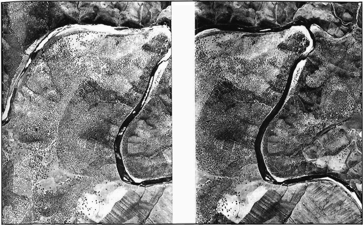
Figura 3.24.- Visión estereoscópica de un tramo del río Agueda, encajado entre las rocas pizarrosas del grupo (111a), y de los relieves característicos de las mismas. Proximidades de la alquería de Marialba (Hoja 525-1). Fragmento obtenido de los fotogramas n os 40.319 y 40.320 de la mencionada Hoja.
