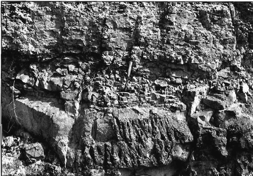
Figura 3.17.- Areniscas del grupo (312a), en las proximidades de la localidad de Canillejas (Hoja 477-1). Pueden observarse dos niveles con distinto grado de fisuración, que indica cambios en la calidad del macizo.
