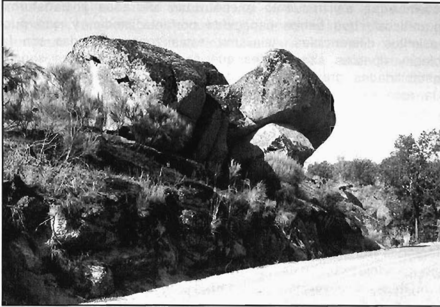
Figura 3.43.- Talud de baja altura realizado en los granitos del grupo (001a). Puede observarse la inestabilidad potencial de las "bolas graníticas", al estar apoyadas en una diaclasa de descompresión que tiene una orientación desfavorable. Proximidades del balneario de Retortillo (Hoja 501-4).
