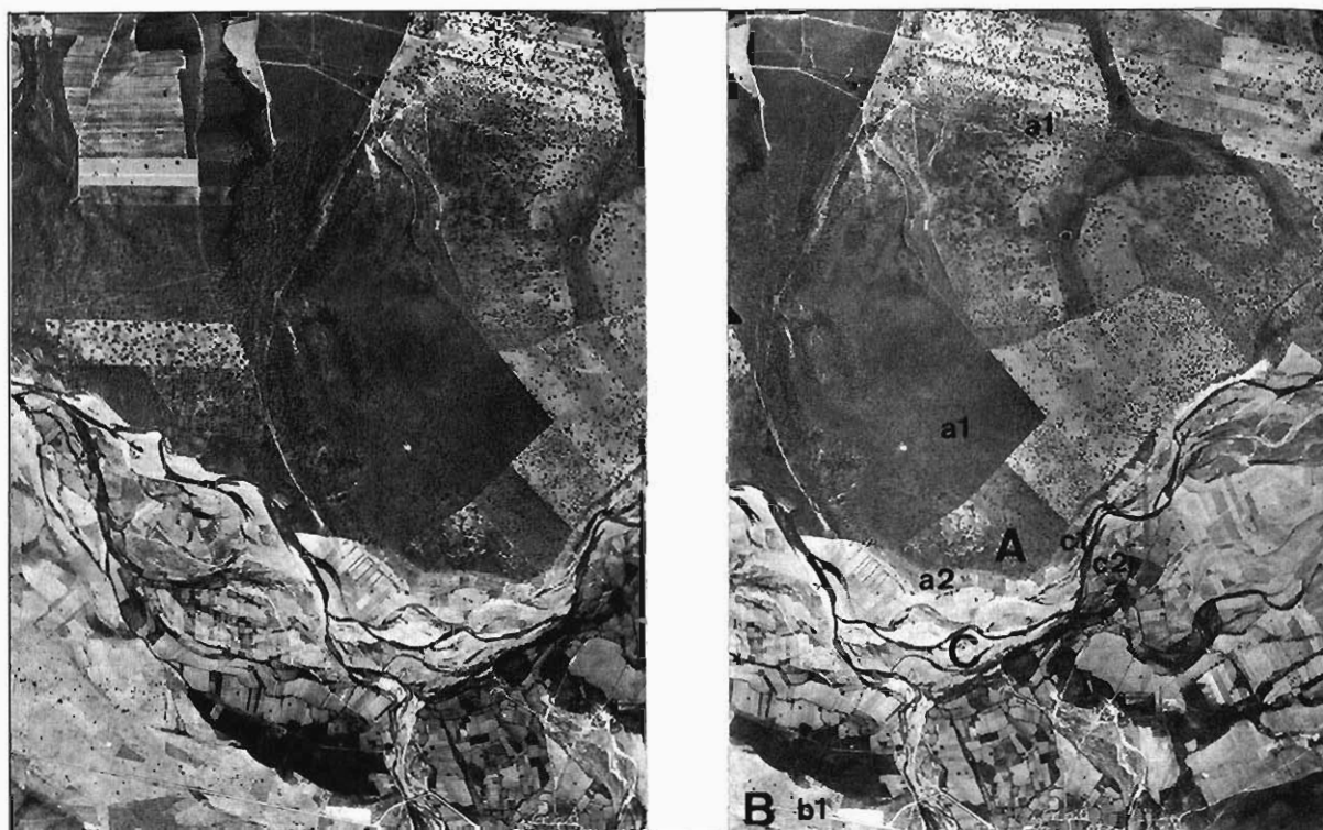
Figura 3.4.- Par estereoscópico parcial de una zona situada al norte de la localidad de Alba de Yeltes (Hoja 501-2), en el paraje denominado "laderas de Tejar". En la Figura: A= margen derecha del río Yeltes, a1= zonas de escorrentía deficiente, y a2= ladera escarpada. B= margen izquierda, y b1= ladera suave. C= cauce actual trenzado del río, c1= desplome del escarpe por erosión, y c2= sedimentación. Fragmento obtenido de los fotogramas n os 5340 y 5341 (vuelo americano) de la Hoja 501-2.
